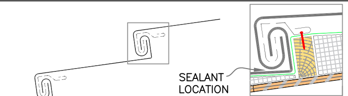
(D) APPLIED BATTEN SEAM
