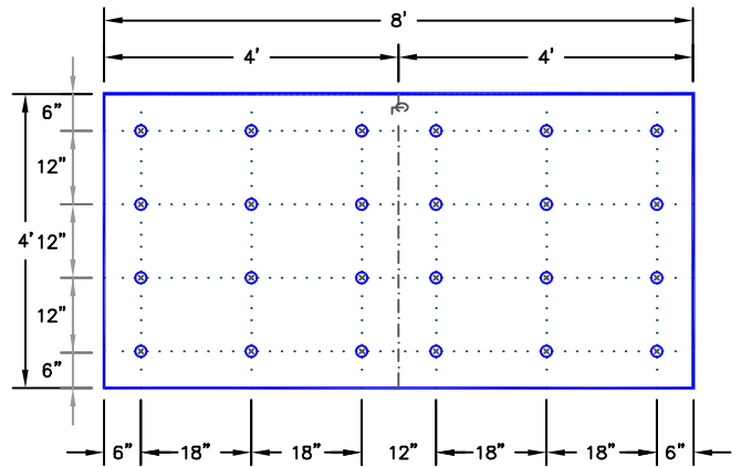
24 FASTENERS PER 4'X8' BOARD
