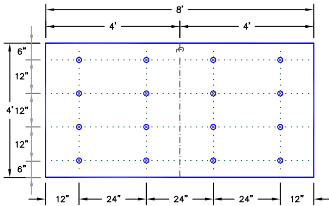
16 FASTENERS PER 4'X8' BOARD
