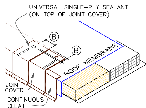
VGC-1.4 VersiTrim Drip Edge Fascia
