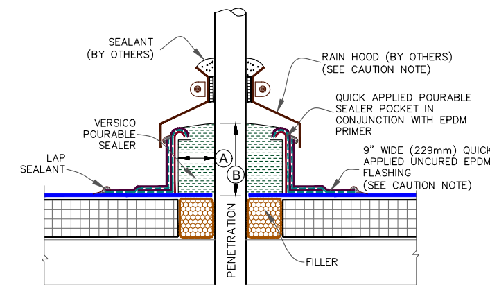
VGC-16 Pourable Sealer Pockets
