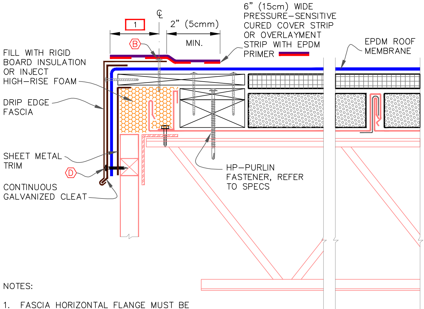
EXISTING FLOATING RAKE EDGE
