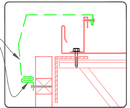
EXISTING FLOATING RAKE EDGE
