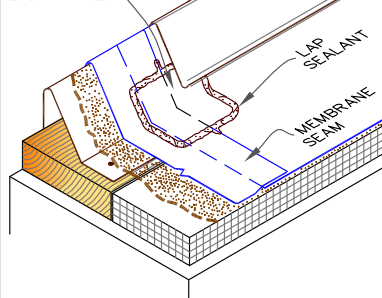
MEMBRANE SEAM AT EDGE
