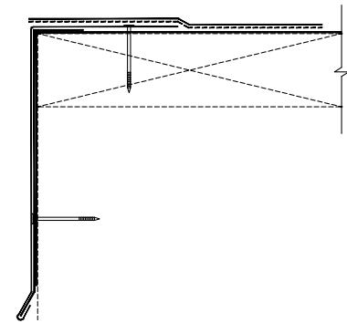
Drip Edge
