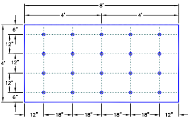
20 FASTENERS PER 4'X8' BOARD
