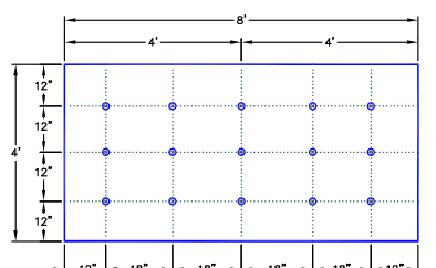
15 FASTENERS PER 4'X8' BOARD
