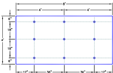
9 FASTENERS PER 4'X8' BOARD
