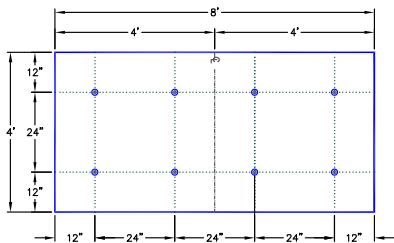
8 FASTENERS PER 4'X8' BOARD
