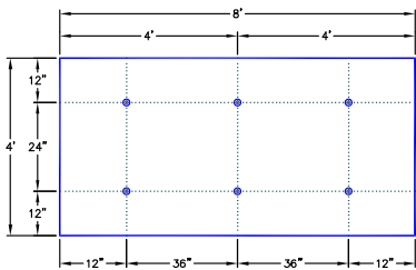
6 FASTENERS PER 4'X8' BOARD
