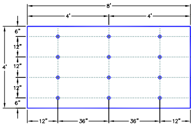
12 FASTENERS PER 4'X8' BOARD
