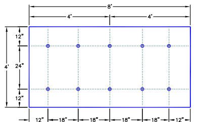
10 FASTENERS PER 4'X8' BOARD
